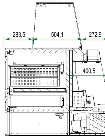
B-B (1:14)
