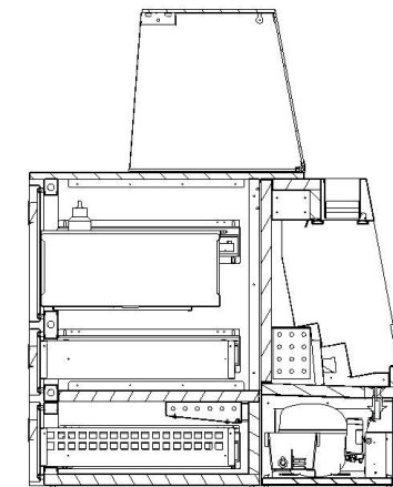
C-C (1:14)
